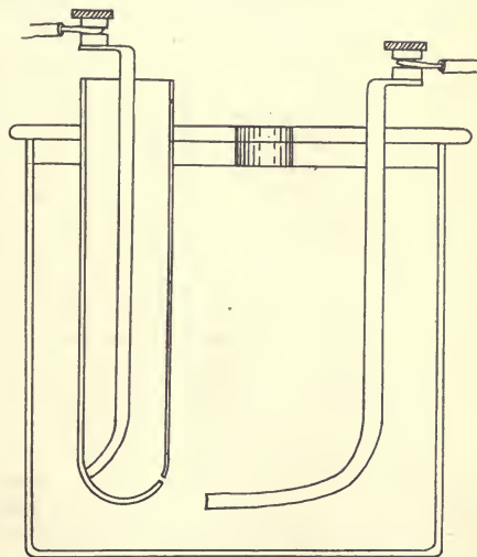
WEHNELT INTERRUPTER.
